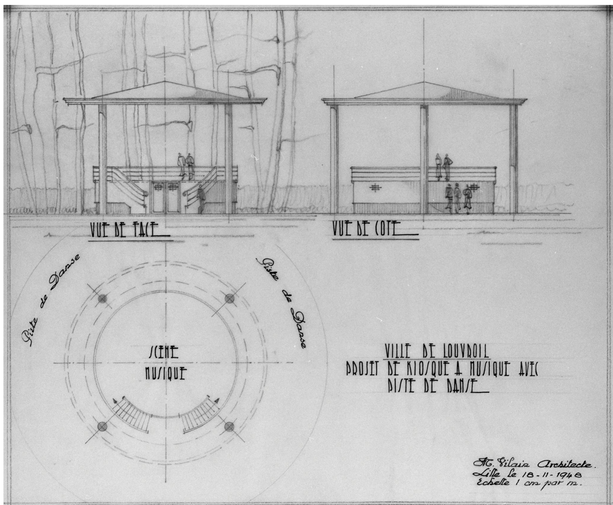
Projet (réalisé) de kiosque à musique avec piste de danse, plan. Vilain (architecte) à Lille, 18 novembre 1948 (AD Nord ; fonds Vilain, 67 J 906).
