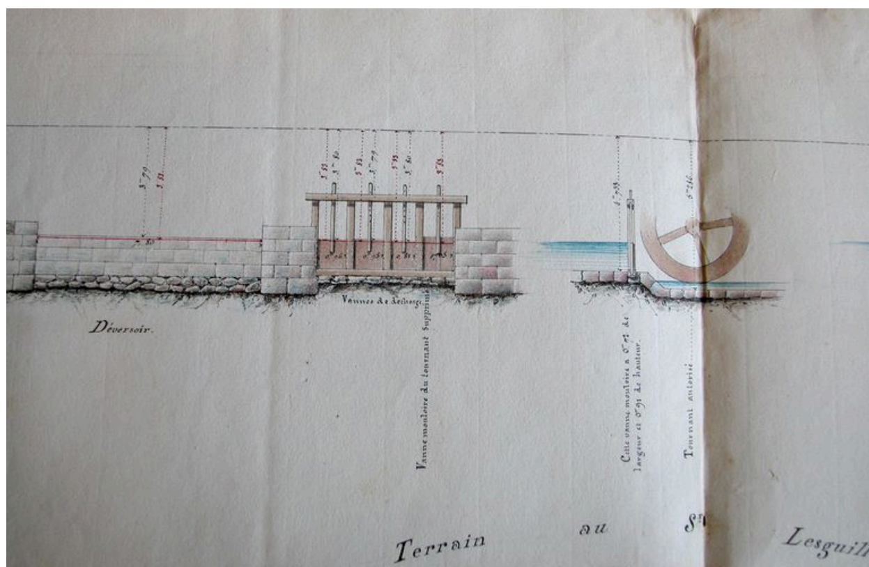
Profil de l'une des roues hydrauliques et du vannage de décharge du moulin Lesguillon, 1831.
