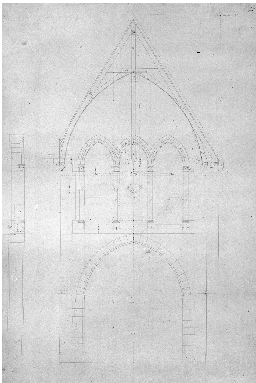
Chapelle, projet de 1856, pignon, coupe sur fenêtre, non signé, non dite. B.M. Boulogne-sur-Mer, mss 535 P, pl. 40.
