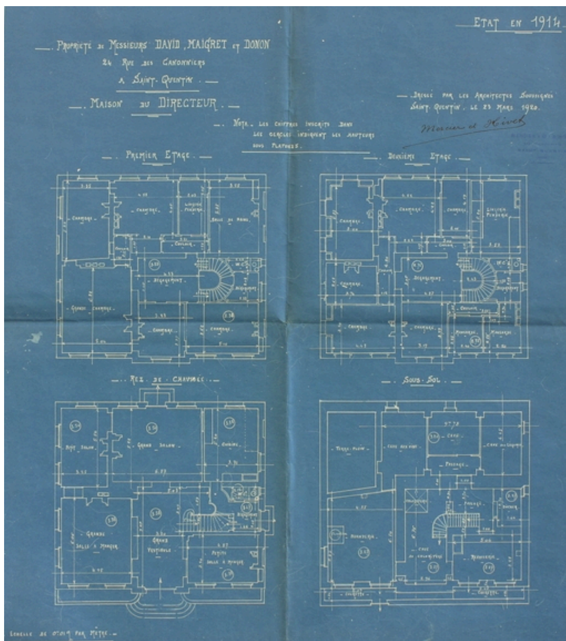
Plans par niveau du logement du directeur, par Mercier et Hivet : état en 1914 (AD Aisne).
