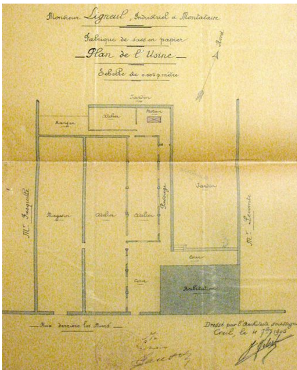
Plan des ateliers et magasins de l'usine de fabrication de sacs en papier, 1905 (AC Montataire ; 304).
