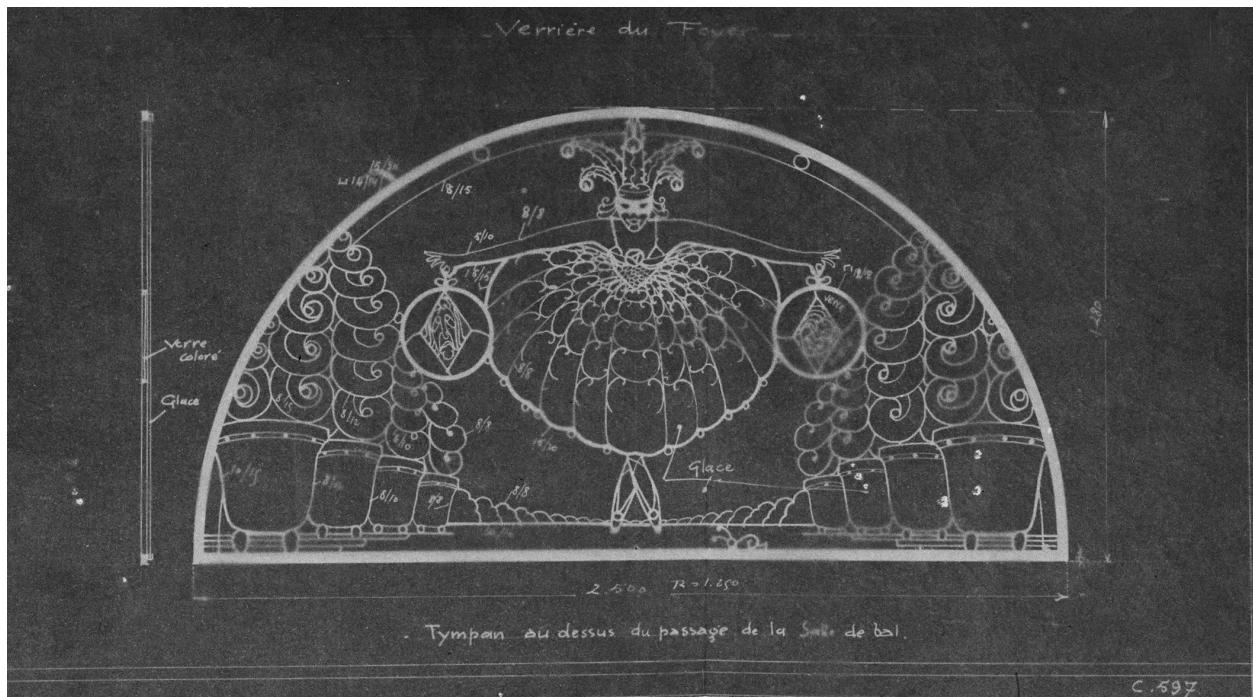
Dessin de ferronnerie pour le tympan du passage du vestibule à la salle de bal. Plan n° C 597 Henri (?) Lafitte (architecte-ingénieur) (AD Nord O396/682).
