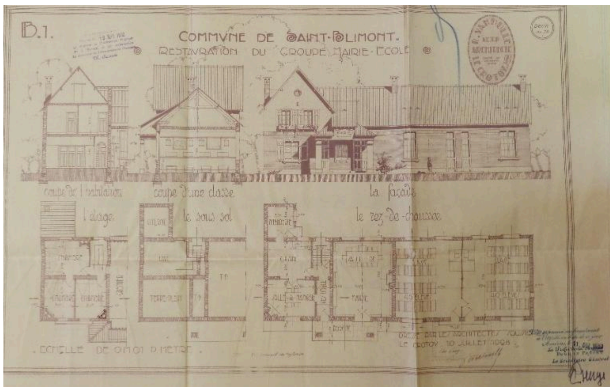
Élévation et plans de sol de la nouvelle école (AD Somme ; 99 O 3366).
