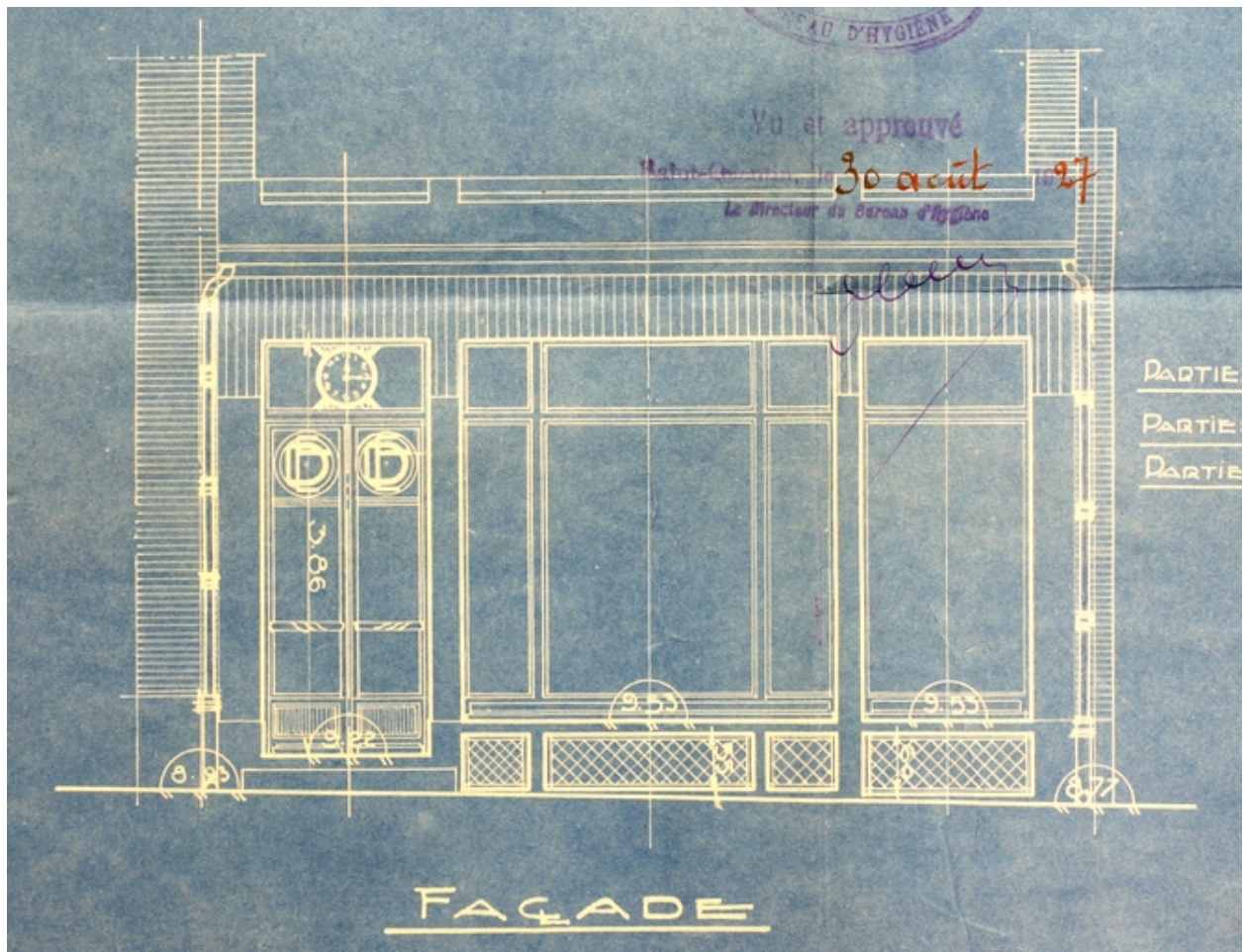
Façade de la salle d'exposition de l'usine (boulevard Gambetta), par Veber et Michau, 1927 (AC Saint-Quentin).
