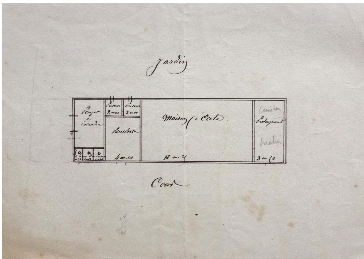
Plan du rez-de-chaussée du bâtiment accueillant l'école de garçons, [entre 1867 et 1880] (AC Pierrefonds ; non coté).
