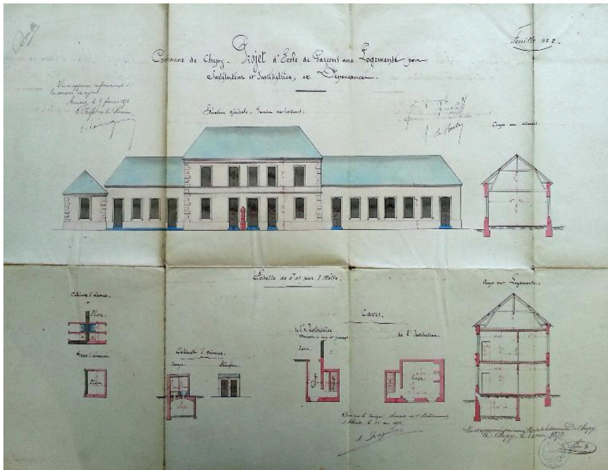
Plans dressés par l'architecte Delignères, 1873 (AD Somme ; 99 O 1145).
