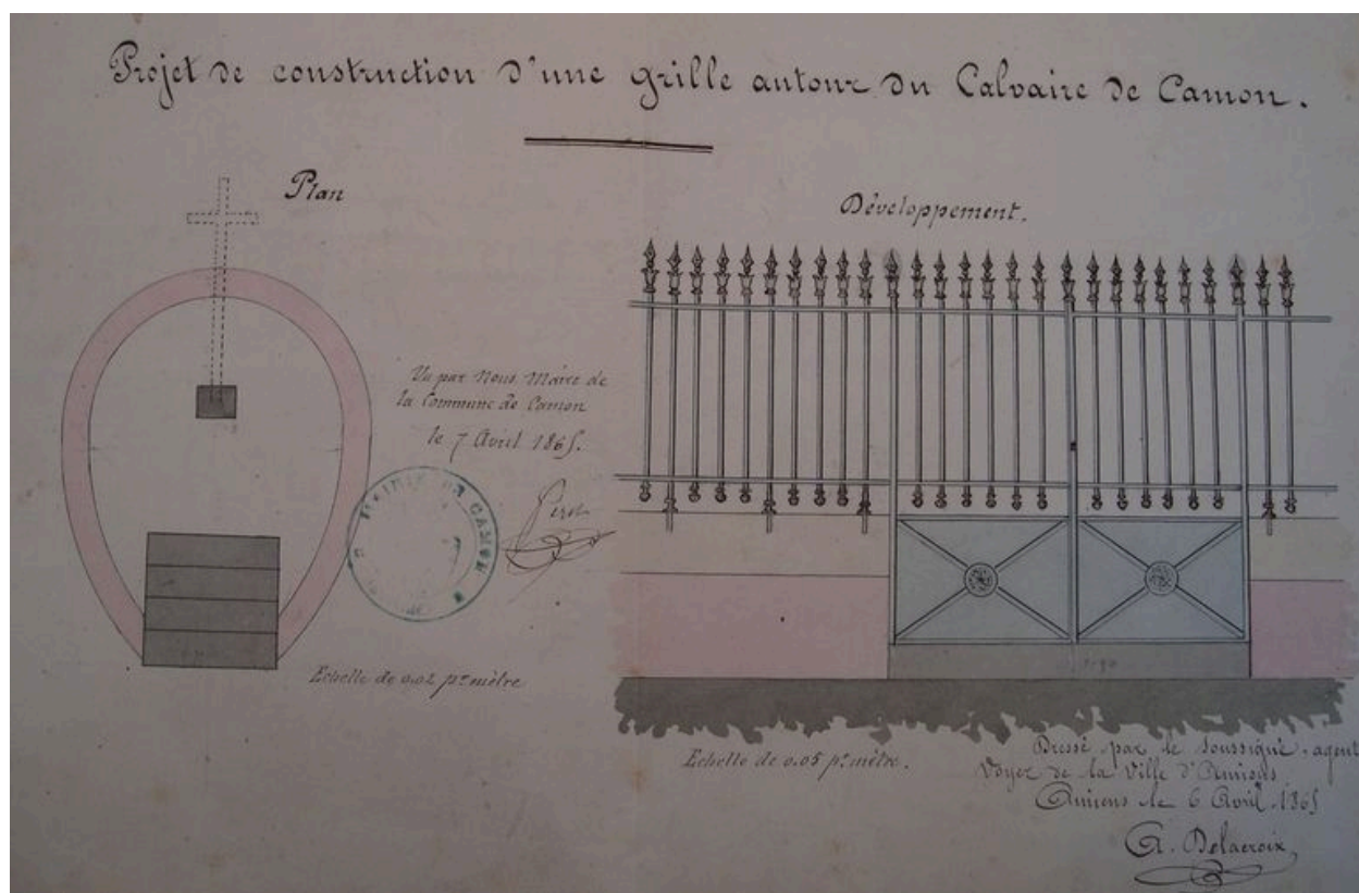
Camon. Projet de construction d'une grille autour du calvaire de Camon, dessin par A. Delacroix agent voyer, 1865. (AD Somme ; 99 O 1008).
