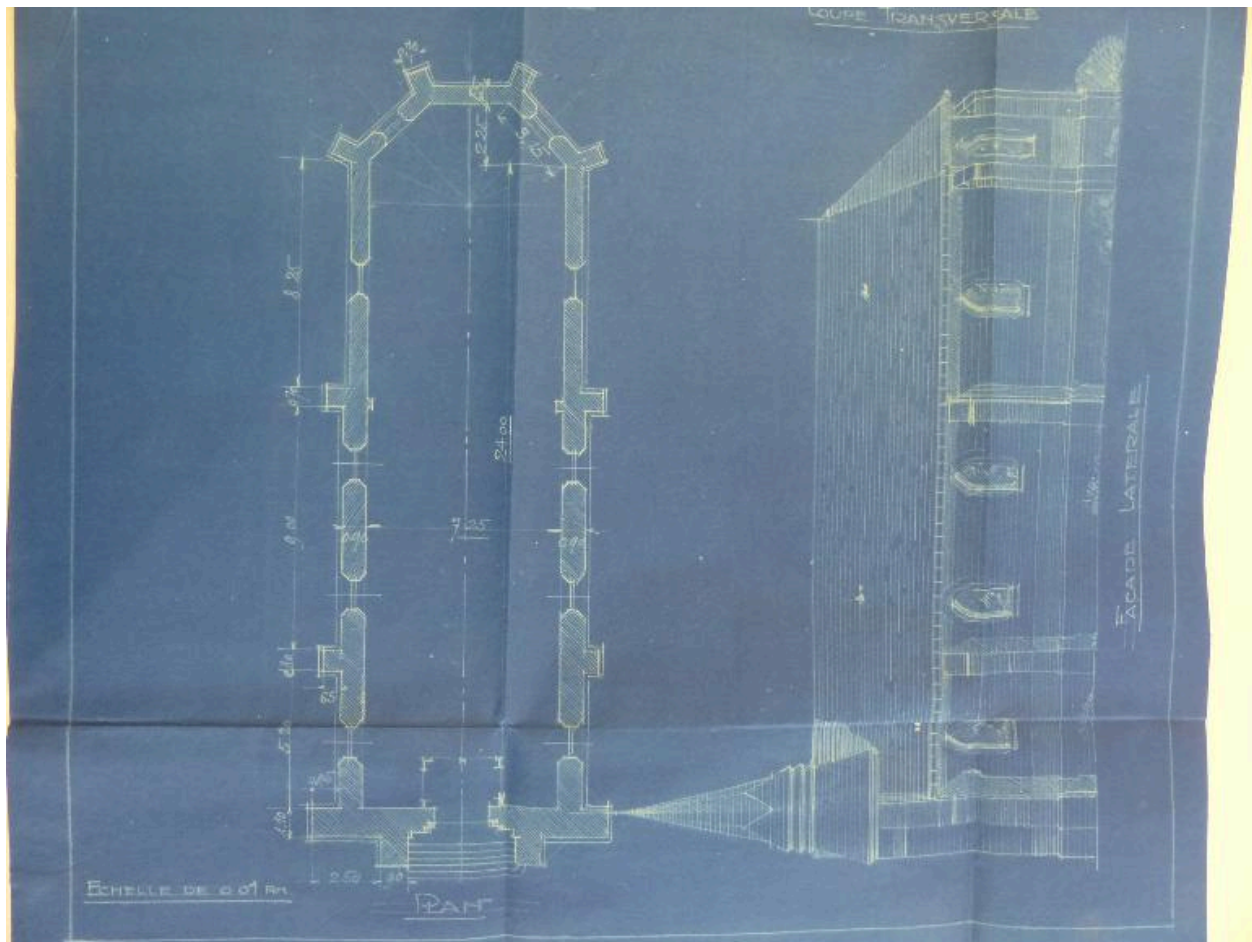
Cachy - Somme. [Ancienne] église, plan au sol et élévation latérale, Louis Duthoit, 1920 (AD Somme ; 10 R 263).
