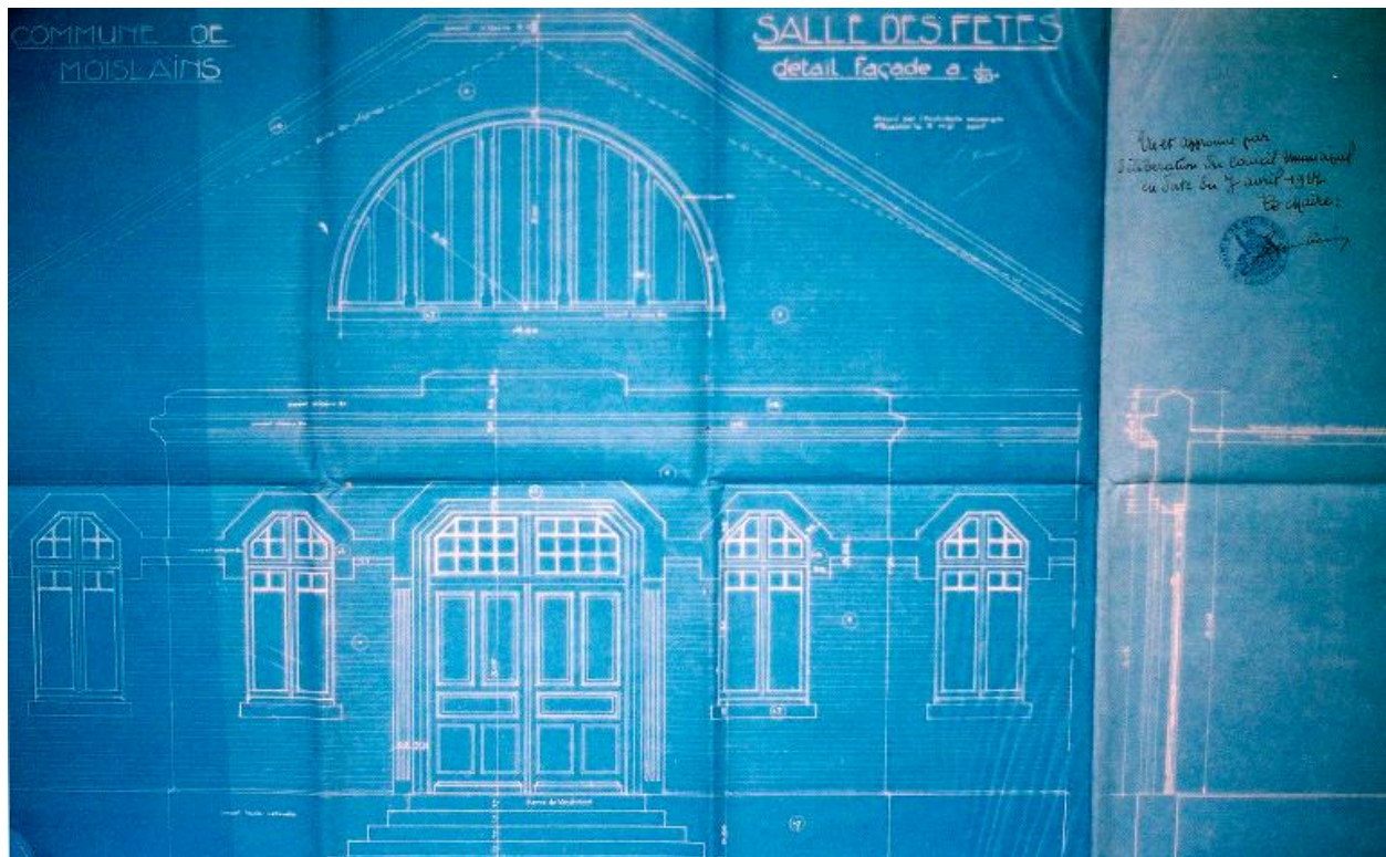
Salle des fêtes, détail de la façade, Pequeux (architecte), 3 mai 1927 (AD Somme ; 99 O 2676).
