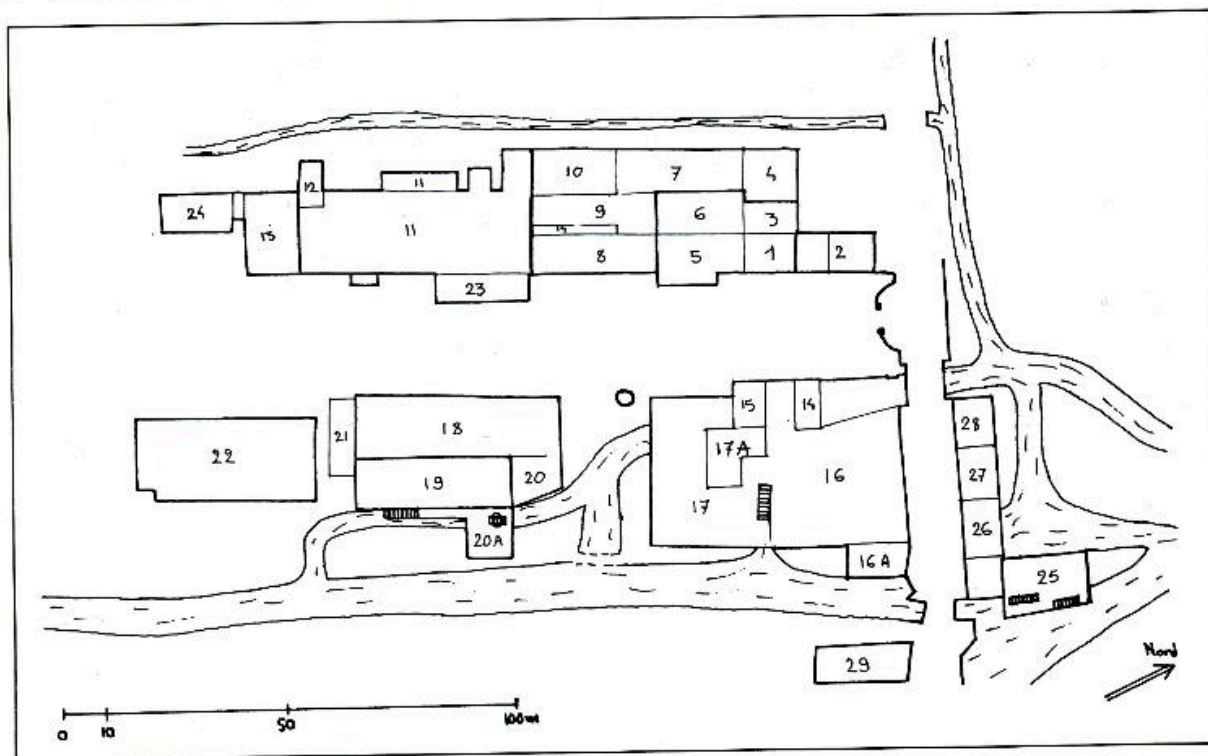
Plan de l'usine en 1943 (Les Cahiers de l'Écomusée, Beauvais, 1987, n°14).
