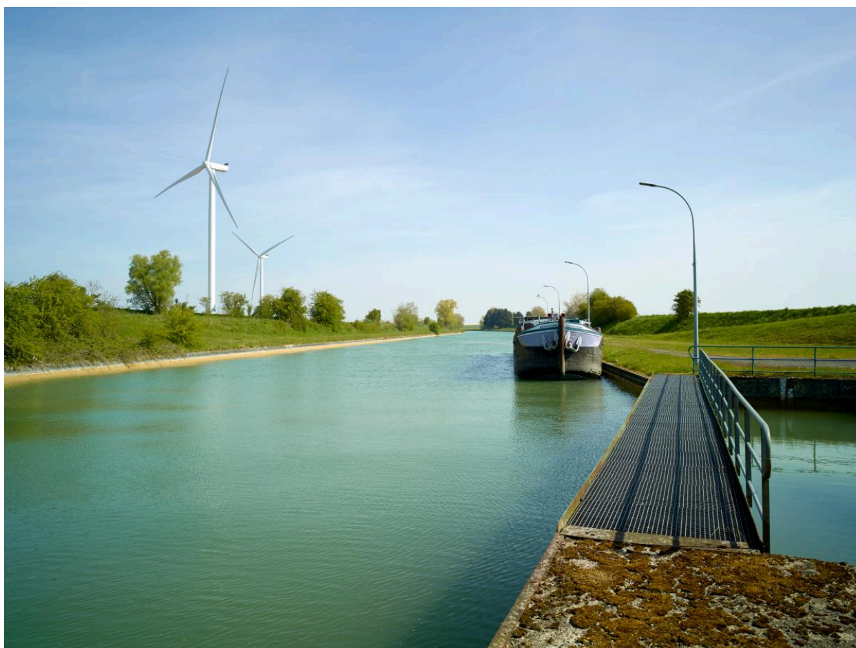
Aval du site d'écluse. Passerelle du bassin de tranquillisation, péniche stationnée.
