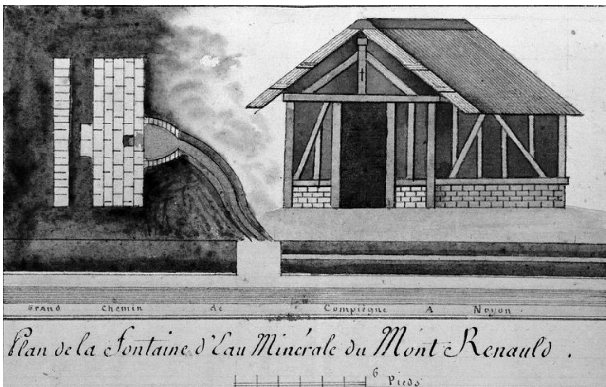
Plan et élévation de la fontaine d'eau minérale du Mont Renault, 1819 (BM Compiègne ; fonds Léré de C. n 58b, f 85).
