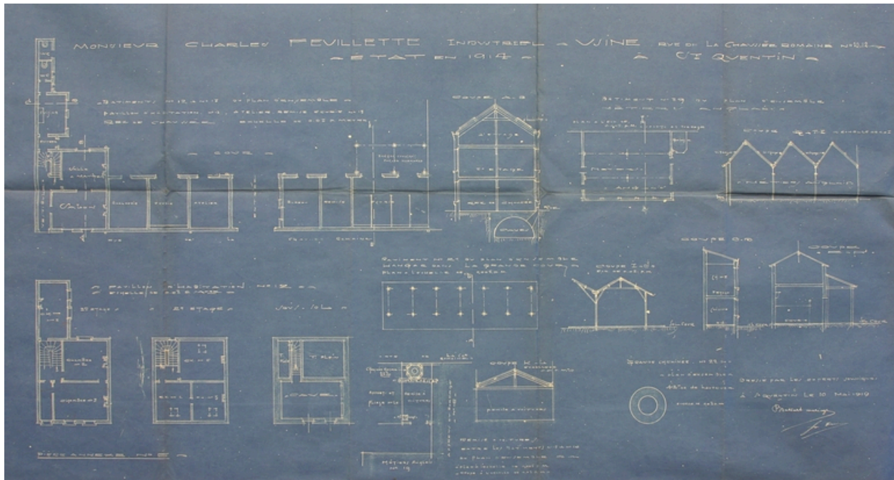
Plan de l'atelier des métiers anglais et de divers autres ateliers en 1914, par Brassart-Mariage, mai 1919 (AD Aisne).
