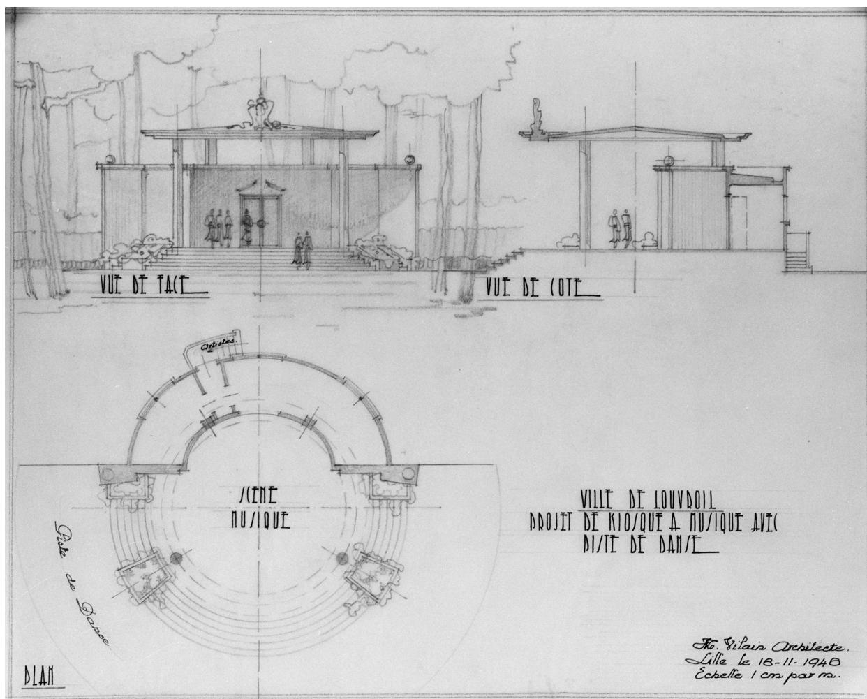
Projet de kiosque à musique avec piste de danse, plan. Lille. Vilain (architecte) à Lille, 18 novembre 1948 (AD Nord ; fonds Vilain, 67 J 906).
