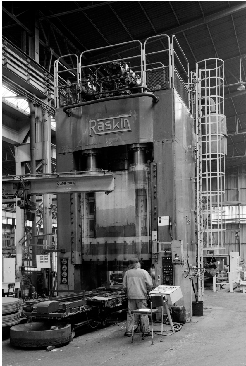
Hall 5 : vue générale de la presse à froid Raskin, 2 000 tonnes, emboutissant des tôles de 1 000 à 1 900 mm.
