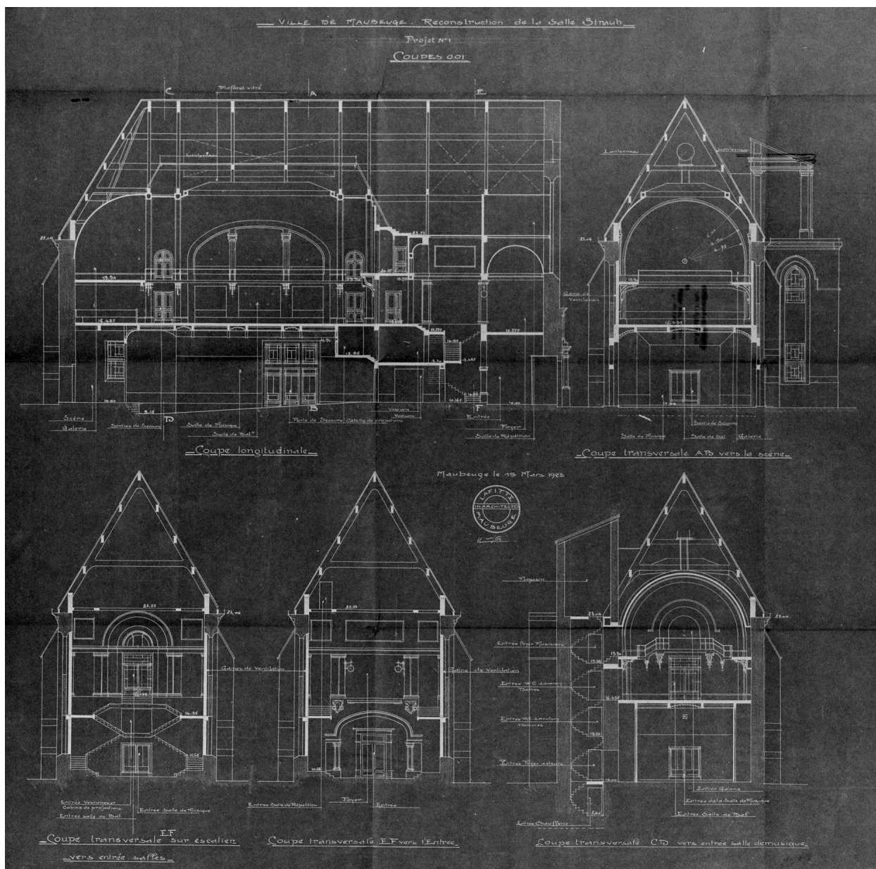
Projet n° 1 de reconstruction de la salle Sthrau, coupes. Plan n° A 735, Maubeuge, 15 mars 1923, par Jean et Henri Lafitte (ingénieurs-architectes) (?) (AD Nord O396/682).
