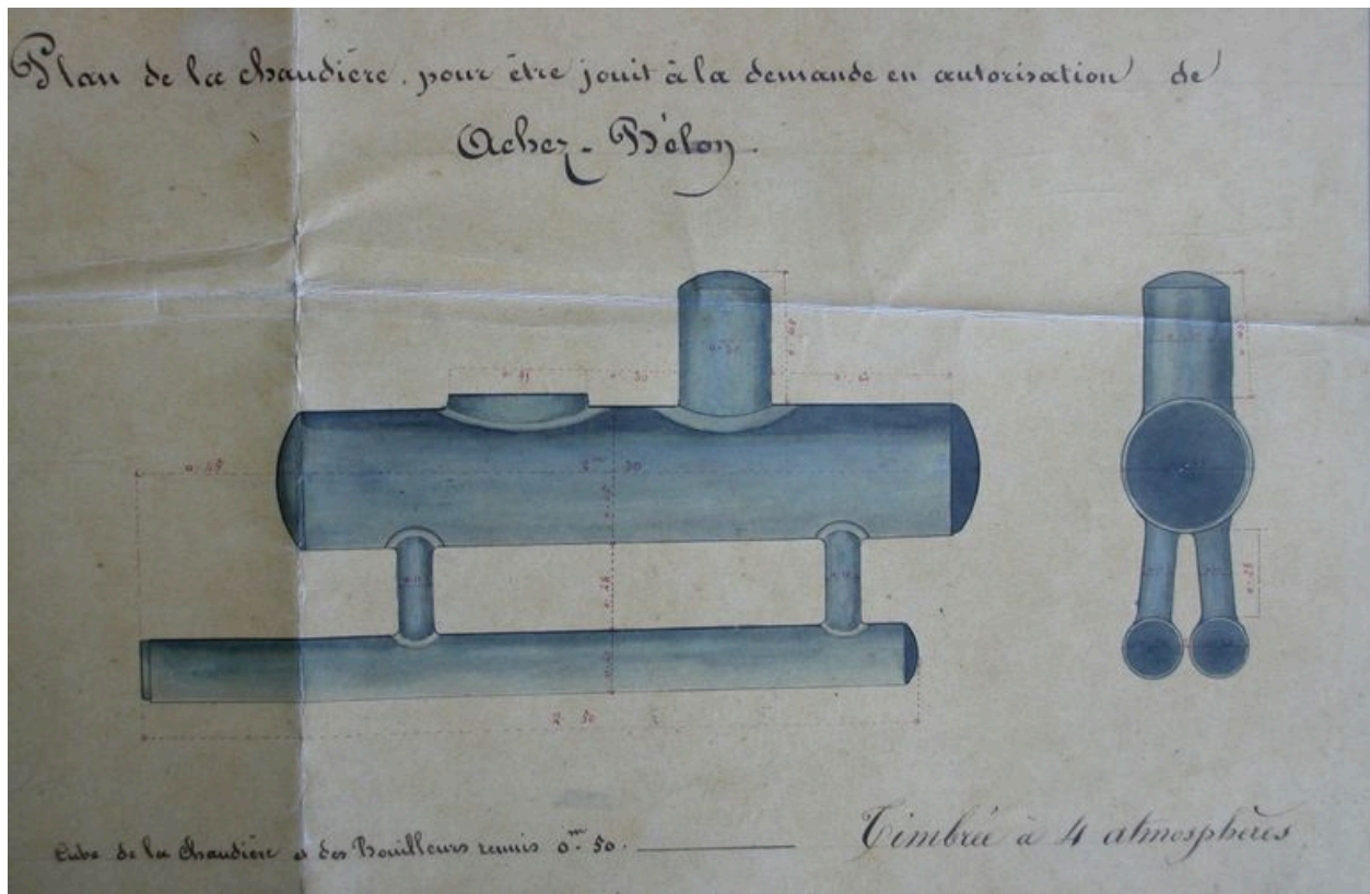
Elévation et coupe de la chaudière à vapeur, annexée à la demande de M. Achez (détail), 1845.
