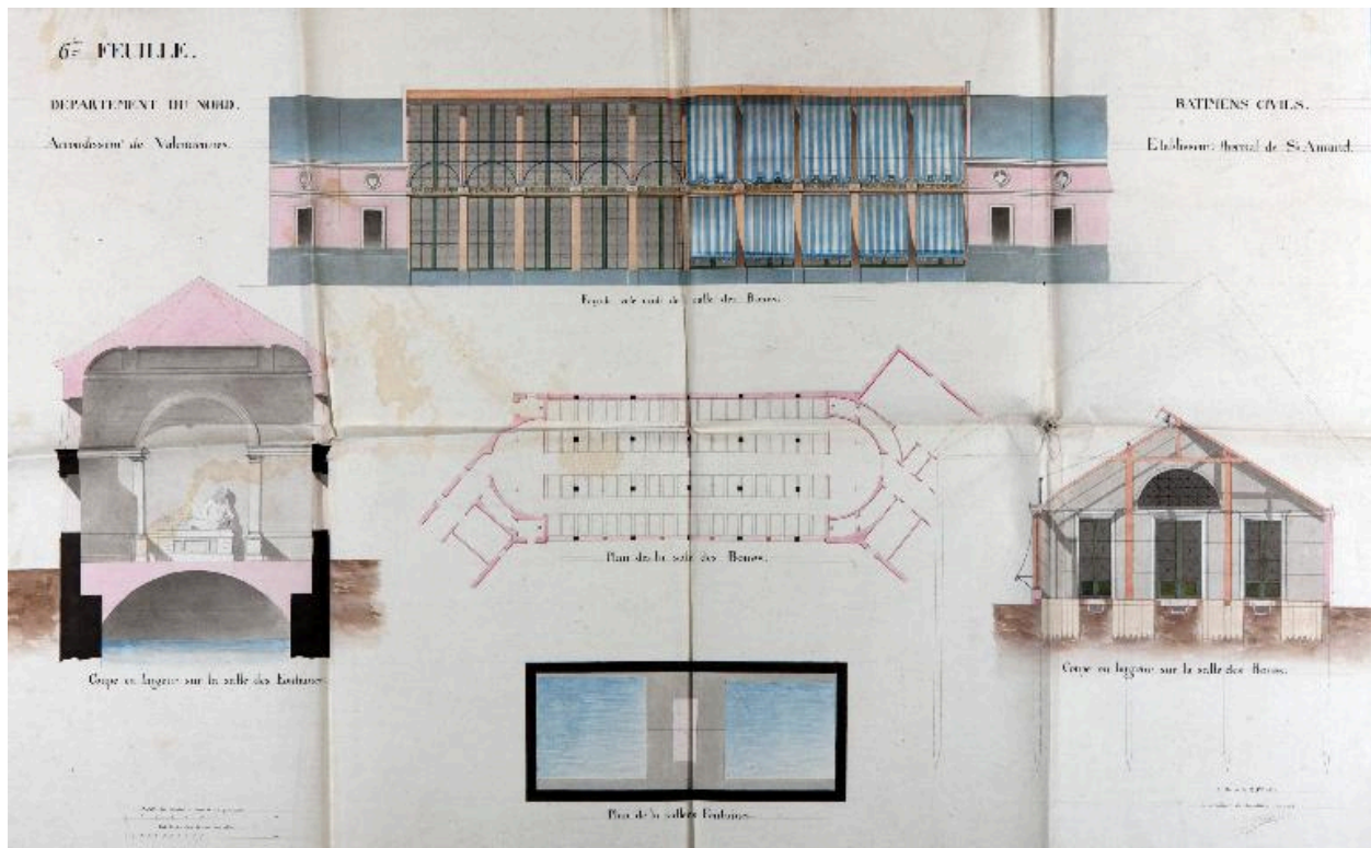
Plan du bâtiment des boues et des fontaines après restauration projetée, 28 septembre 1830, Malet architecte départemental (AD Nord, 4N 553).
