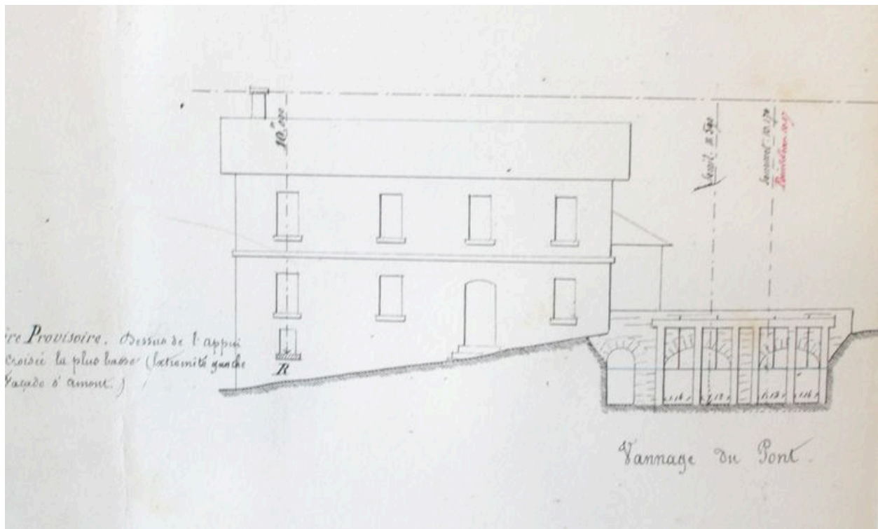
Élévation du moulin, 2 juillet 1856 (AD Oise ; 7Sp 142).
