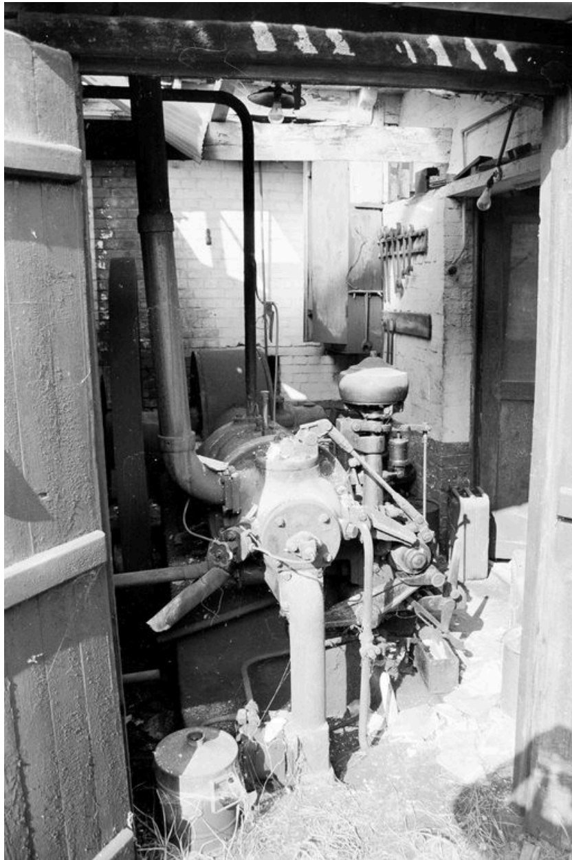
Moteur à pistons à combustion (machine à pression d'huile) : vue de face.
