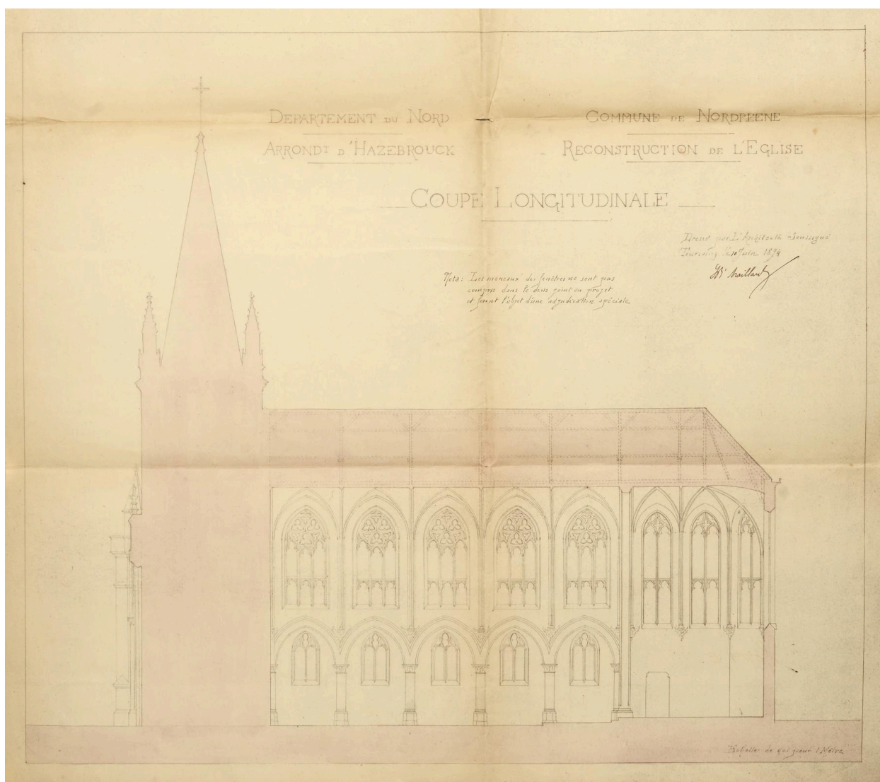
Reconstruction de l'église de Noordpeene. Coupe longitudinale. Dressée par l'architecte Maillard le 10 juin 1894 (AD Nord : 2 O 437/18).
