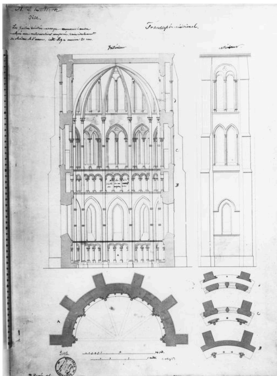
Bras sud du transept, projet de restauration. Plans et élévations, par D. Ramée, 1842.
