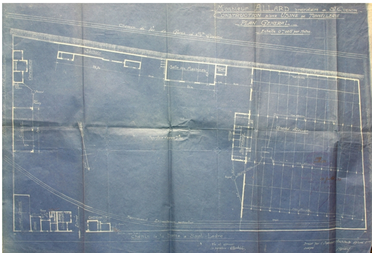
Plan de l'usine, par R. Viard, 1923 (AC Saint-Quentin).
