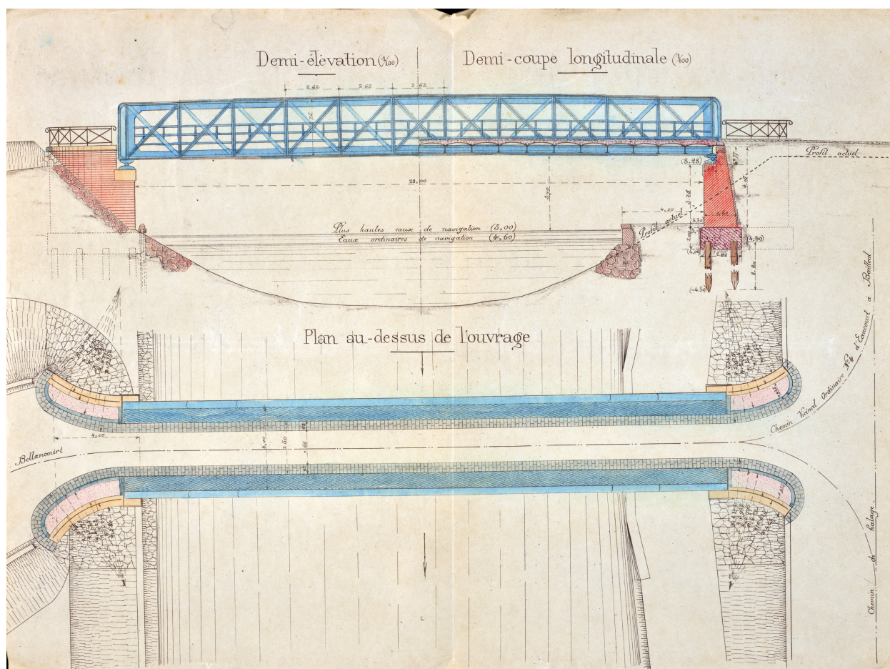
Plan, élévation et coupe, pont d'Eaucourt-sur-Somme, 27 Juillet 1905 (AD Somme ; 99 O 1483).
