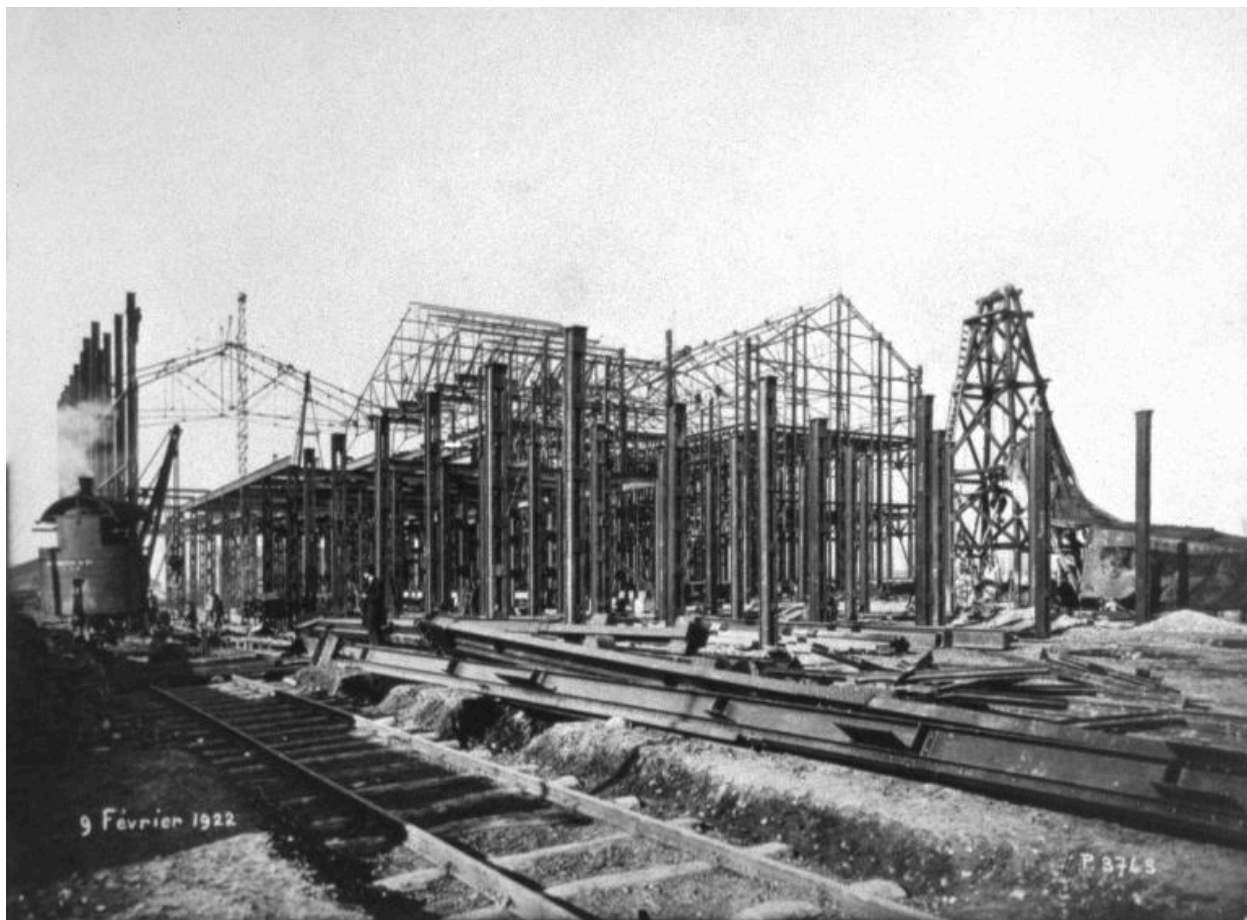
Montage de la structure métallique de la sucrierie, 9 février 1922 (Archives privées de l'entreprise).
