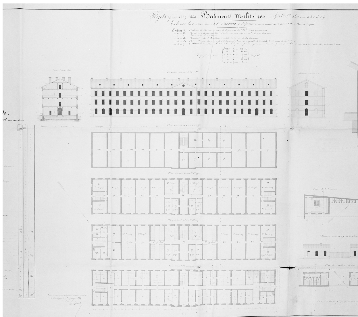
Bâtiment principal : plans, coupe, façade, 1859. A. Génie Vincennes, Boulogne, art. 8, section 1, carton 9.
