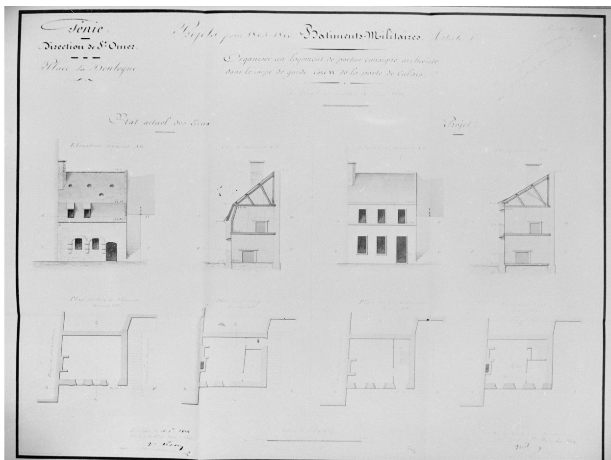
Etat des lieux en 1864, projet d'aménagement A. Génie Vincennes, Boulogne, art. 8, sect. 1, cart. 9.
