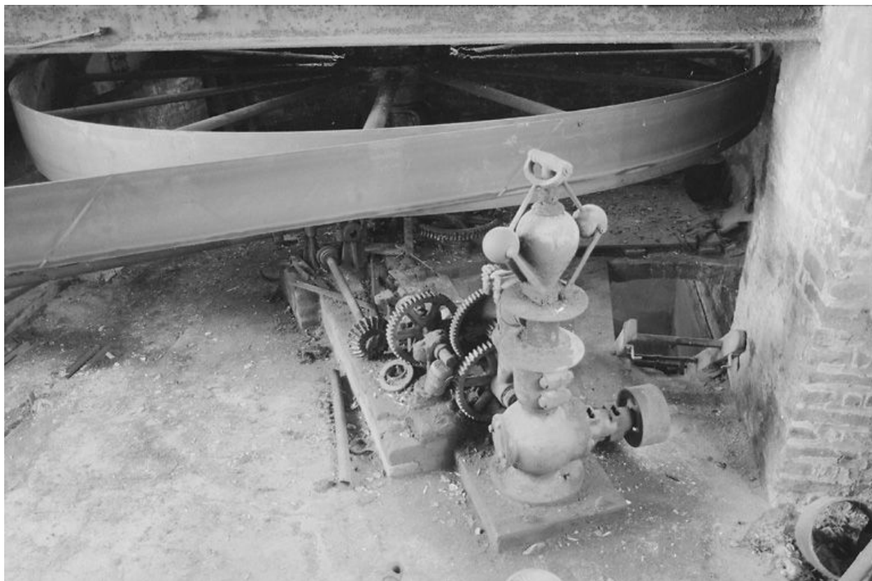
Régulateur.
