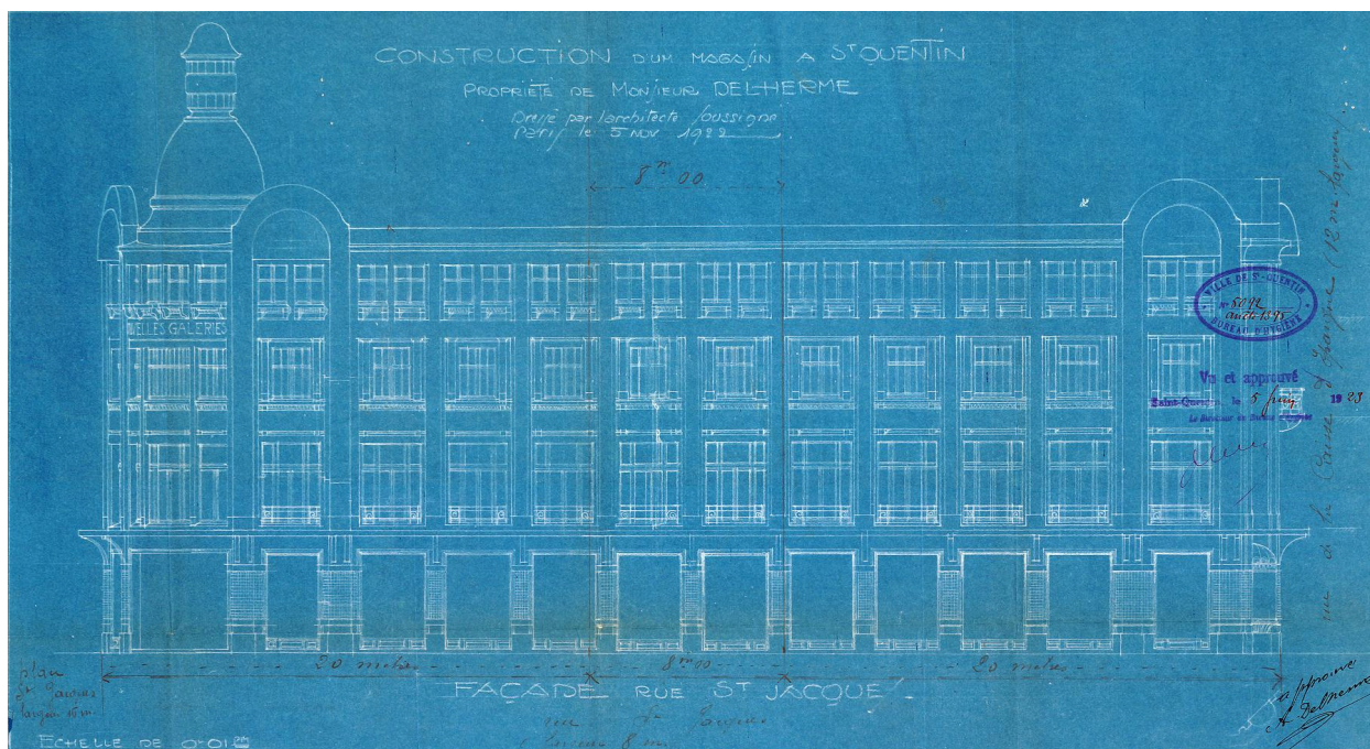
Élévation de la façade est, rue Saint-Jacques, 5 novembre 1922 (Archives municipales de Saint-Quentin).
