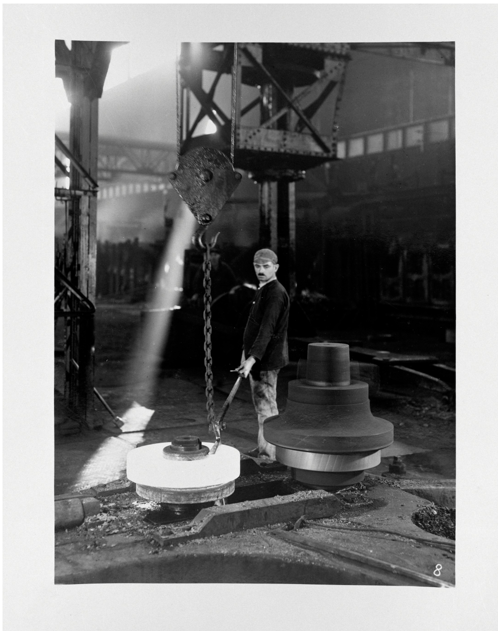
Laminoir à bandages. Photographie ancienne, auteur inconnu, sans date (coll. part.).
