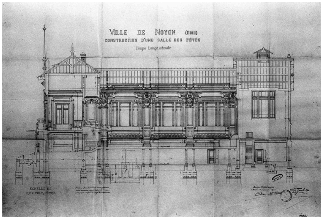
Coupe longitudinale, projet par C. Letrosne, 1903 (AD Oise ; série O).
