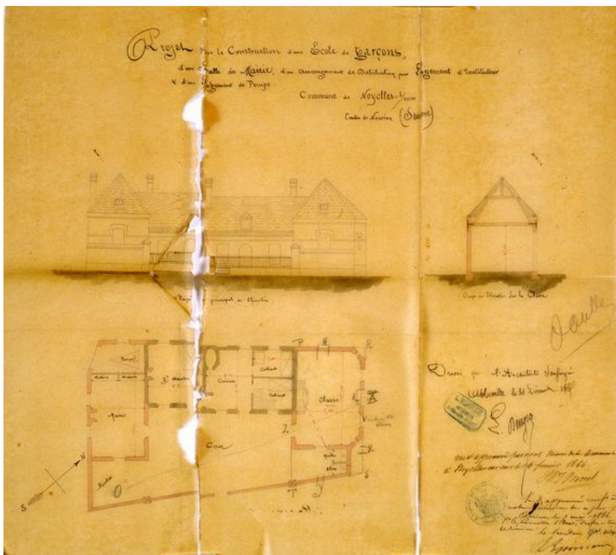
Projet pour la construction de l'école des garçons, d'une salle de mairie, d'un arrangement de distribution pour le logement de l'instituteur et d'un logement de pompe dressé par l'architecte soussigné Dingeon en 1865.
