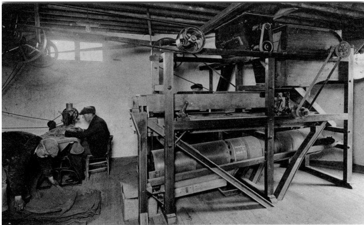
Léon LEGLAND FLINES-LEZ-RACHES (Nord) 8. Appareils pour le nettoyage des trèfles et luzernes et Repriseuse de Sacs
