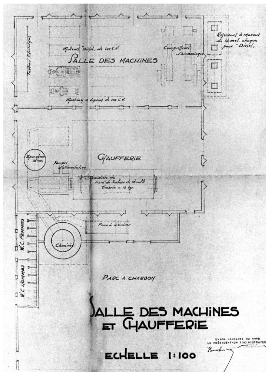
Plan de la salle de chaufferie et des machines (sans date).
