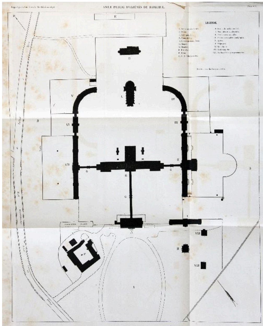
Plan-masse général gravé avec indication du projet de construction d'un second bâtiment dit pavillon d'angle placé en symétrie par rapport au premier, 1874 (AD Nord).
