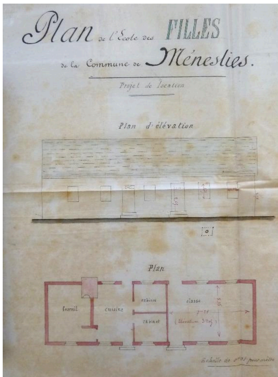
Plan au sol et élévation de l'ancienne école des filles, 1881 (AD Somme ; 99 O 2564).
