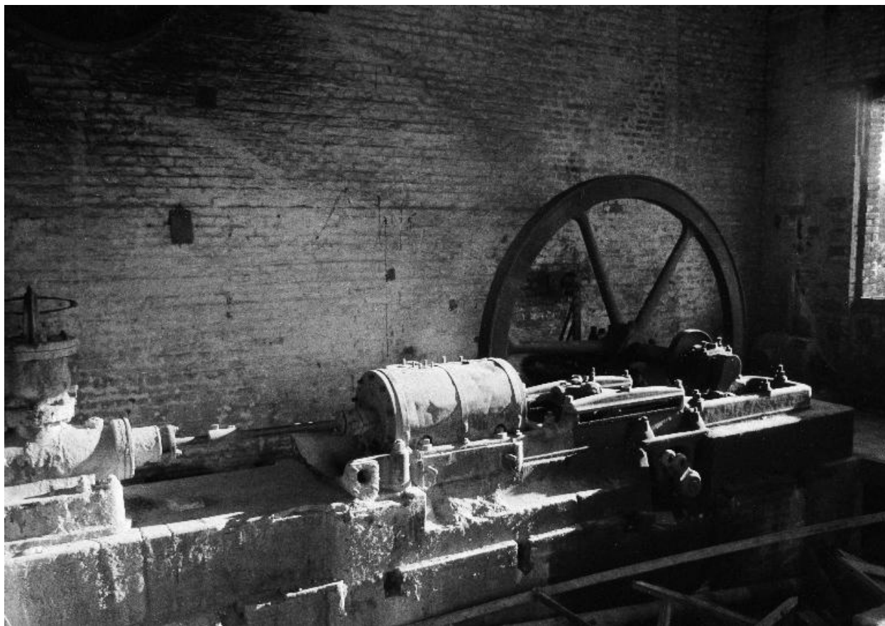
Salle des machines, rue du 19e BCP. Machine à vapeur.
