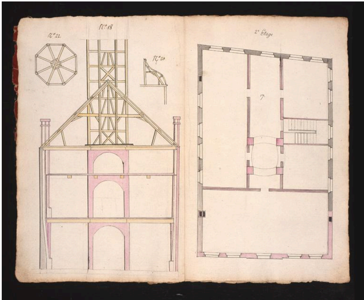
Coupe transversale et plan du 2e étage de l'hôtel de ville de Vervins : projet de réhabilitation non suivi d'exécution, vers 1820.
