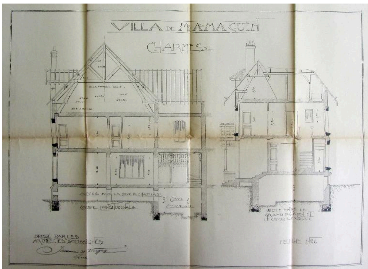
Coupes longitudinale et transversale de la villa de M. A. Maguin, [1912] (AD Aisne ; 15 R 772).
