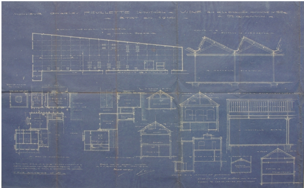
Plan de l'atelier de blanchiment (restauré), de la salle des machines, de la chaufferie (détruits), en 1914, par Brassart-Mariage, mai 1919 (AD Aisne).
