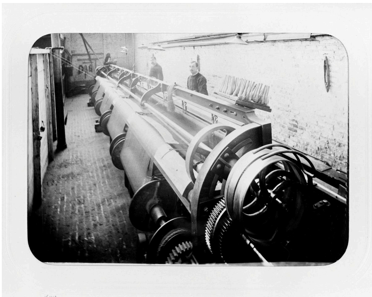
Métier à tisser de 8,30 m. Photographie de J. David, 1897 (AP Hacot et Colombier).
