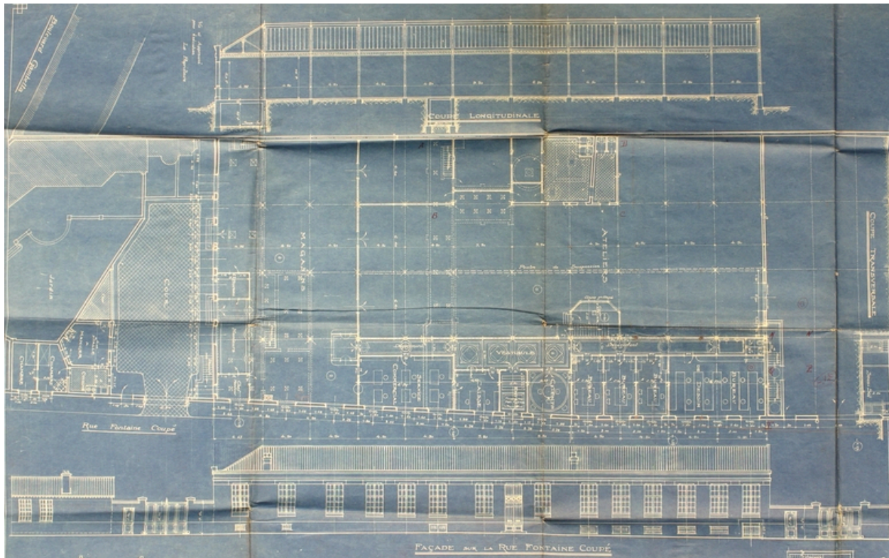
Plan, coupe longitudinale et élévation sur rue des ateliers, par Veber et Michau, 1920 (AC Saint-Quentin).
