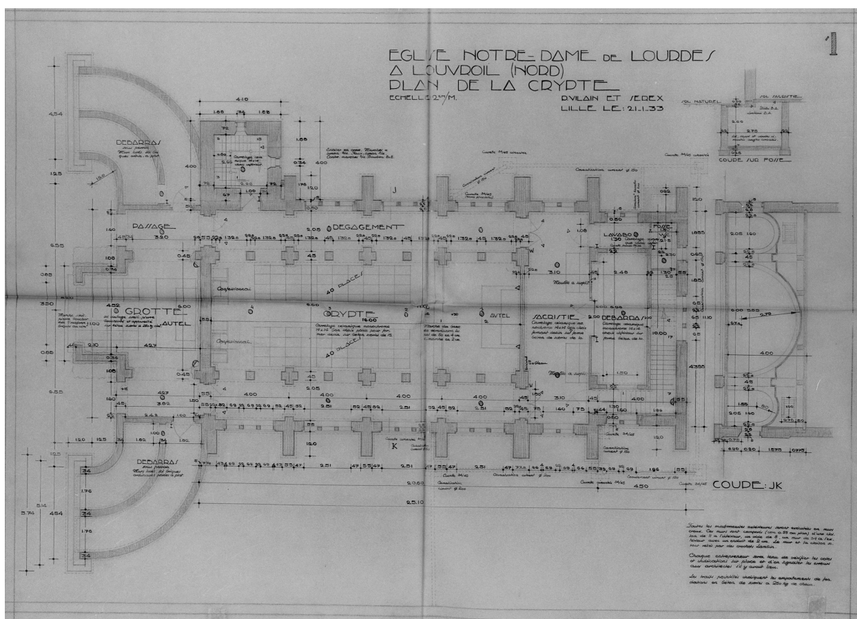
Projet retenu, plan de la crypte. Crayon sur calque des architectes Paul Vilain (1860-1933) et Charles-Paul Serex (1899-1978), Lille, 21 janvier 1933 (AD Nord ; fonds Vilain, 67J903).
