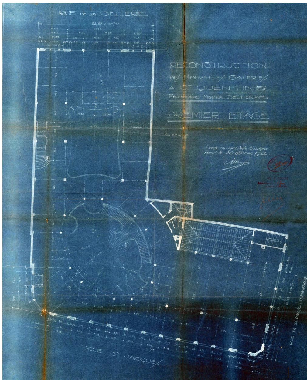
Plan du premier étage des Nouvelles Galeries, 5 novembre 1922 (Archives municipales de Saint-Quentin).
