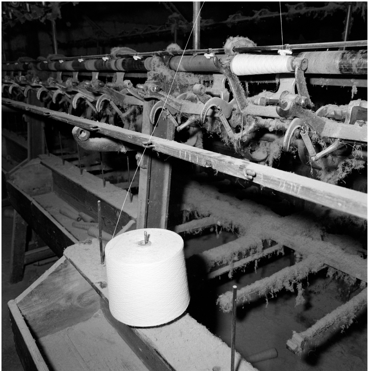
Bobinoir (Cornard, Marcq-en-Barœul). Détail.
