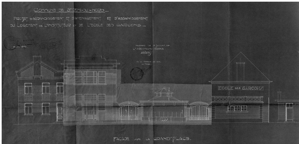
Projet d'agrandissement et d'aménagement du logement de l'instituteur et de l'école des garçons de Saint-Rémy-du-Nord. Élévations sur la Grand'Place. Plan d'Adolphe Danis (1886-1969), 1931 (AD Nord, série O ; 542/81).
